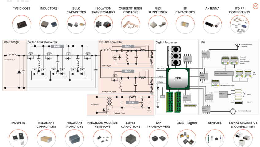
圖二、國巨被動元件在伺服器中的應用
